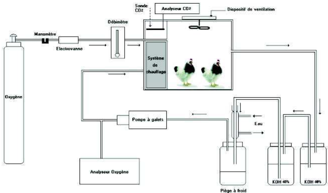
Schéma 3 : Dispositif expérimentale pour la mesure des gaz respiratoires
