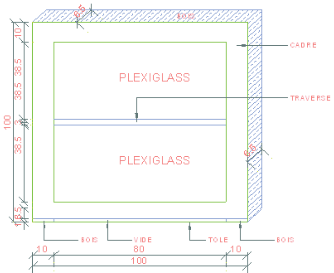
Figure 7 : Caractéristiques de la paroi latéral 2
