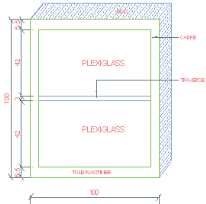
Figure 9 : Caractéristiques de la paroi latéral 4
