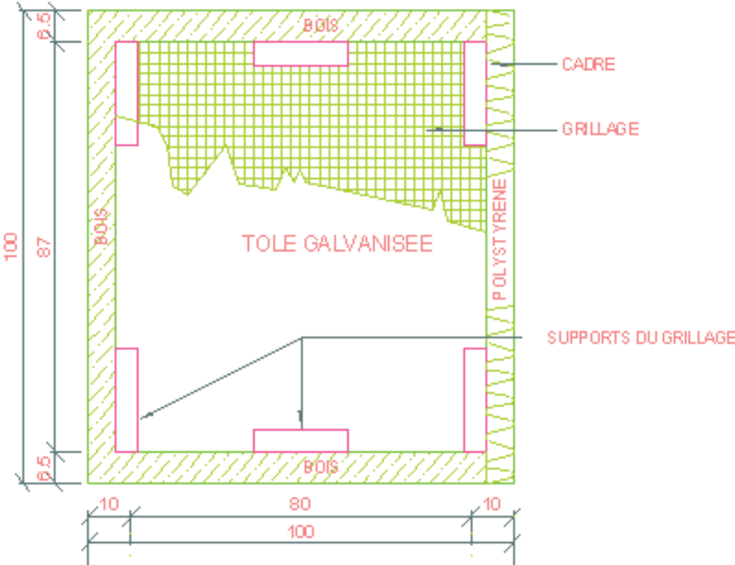
Figure 10 : Caractéristiques du plancher de la chambre respiratoire
