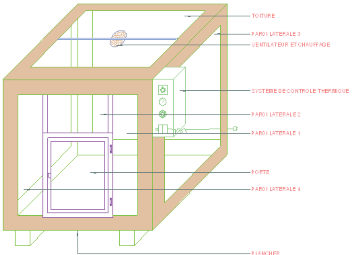
Figure 5 : Vue en perspective de la chambre respiratoire
