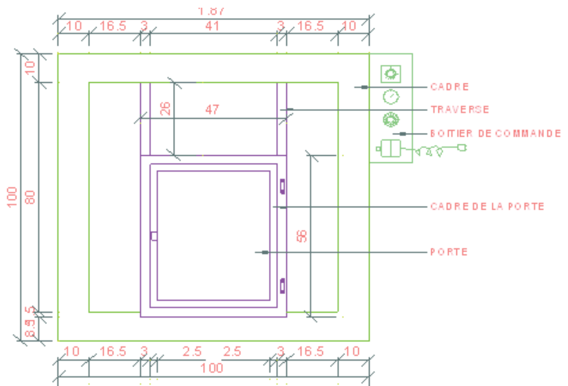
Figure 6 : Caractéristiques de la paroi latéral 1
