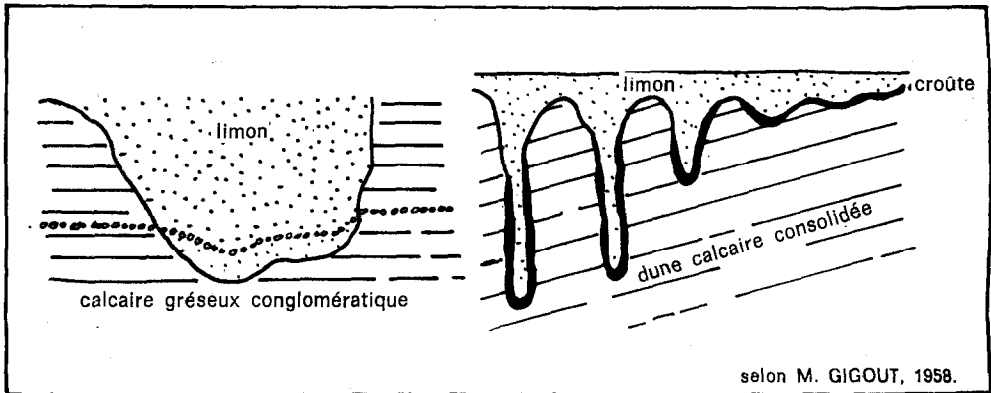
Formation du limon rouge « in-situ » par lessivage du calcaire accumulé en croûte zonaire dans les lapiez.
